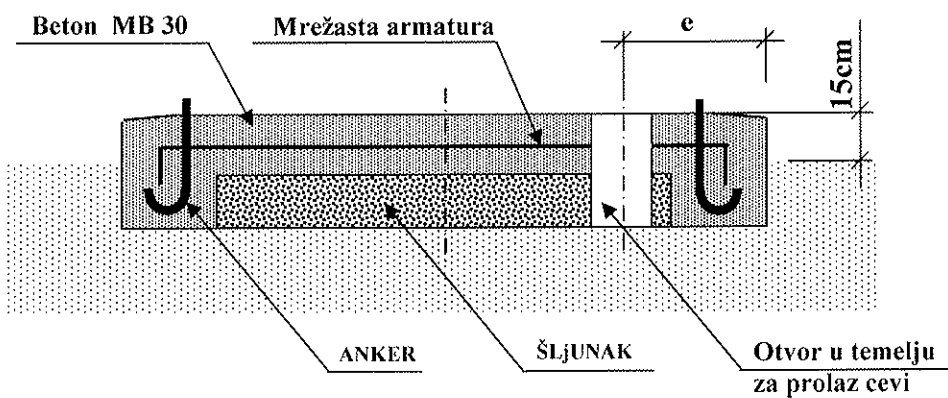
PRESEK B-B
