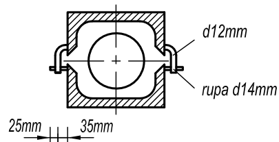
PRESEK A-A
