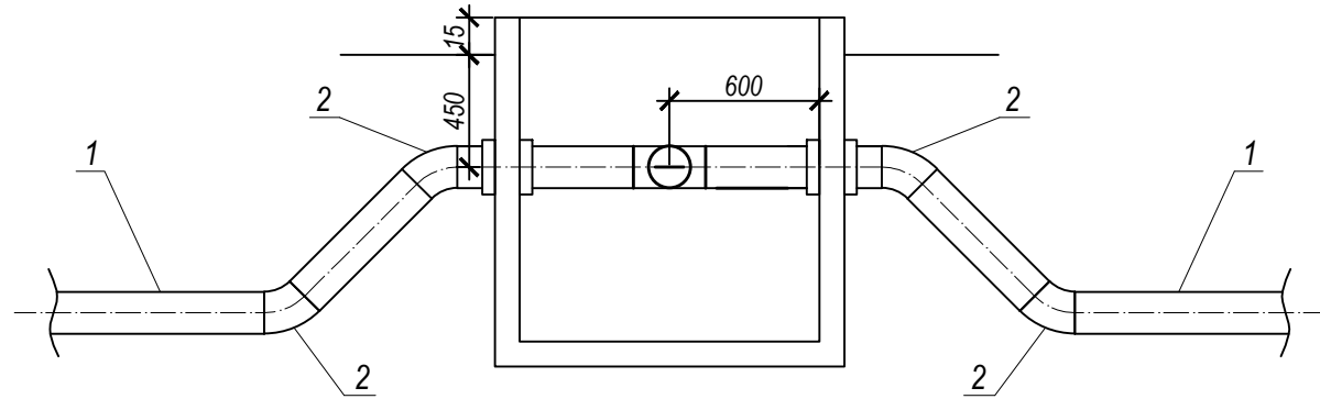
PRESEK A-A
