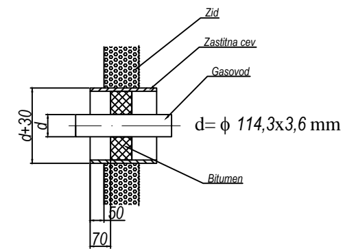
DETALJ "A"
