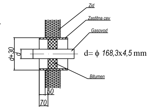
DETALJ "A"
