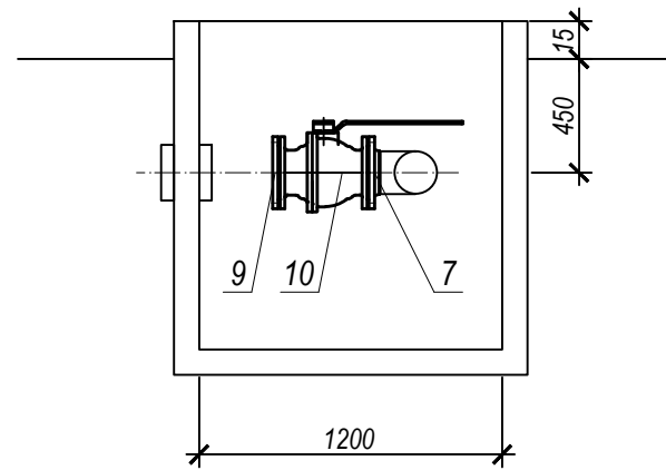
PRESEK B-B
