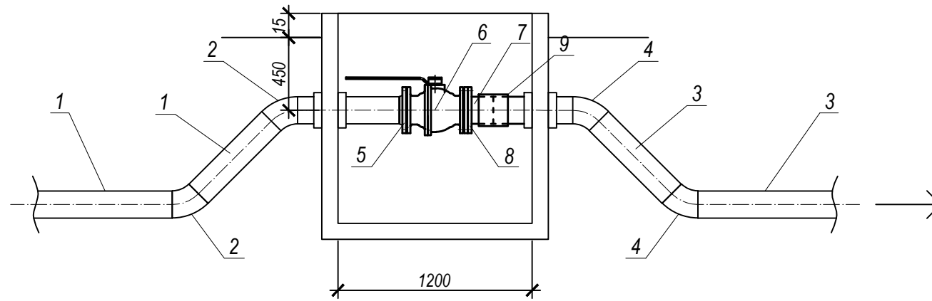
PRESEK A-A
