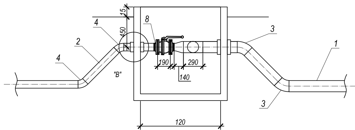
PRESEK A-A
