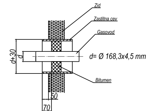
DETALJ "A"
