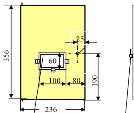
DETALJ VRATA
