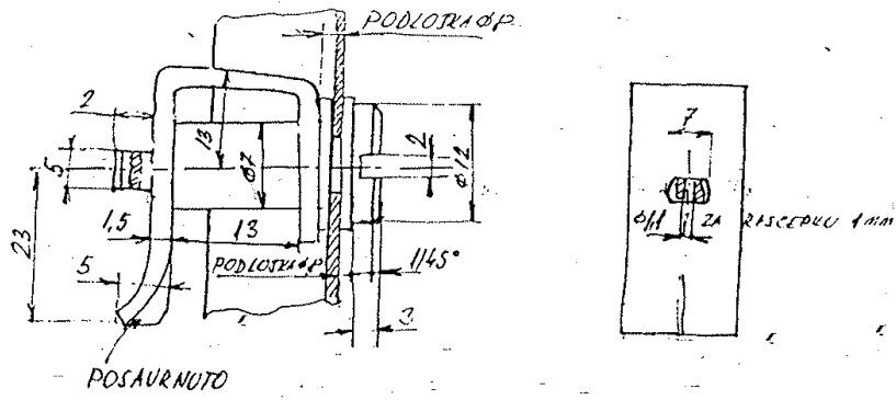
ДЕТАЛ "C"
