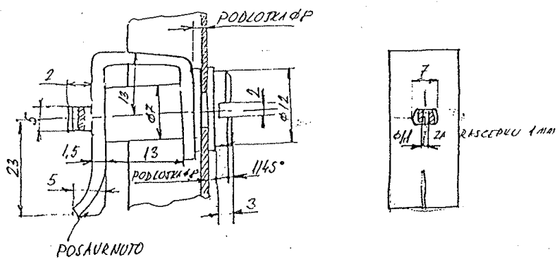
ДЕТАЛЈ "C"
